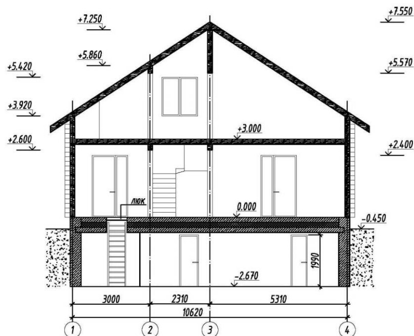
Разрез 2-2
