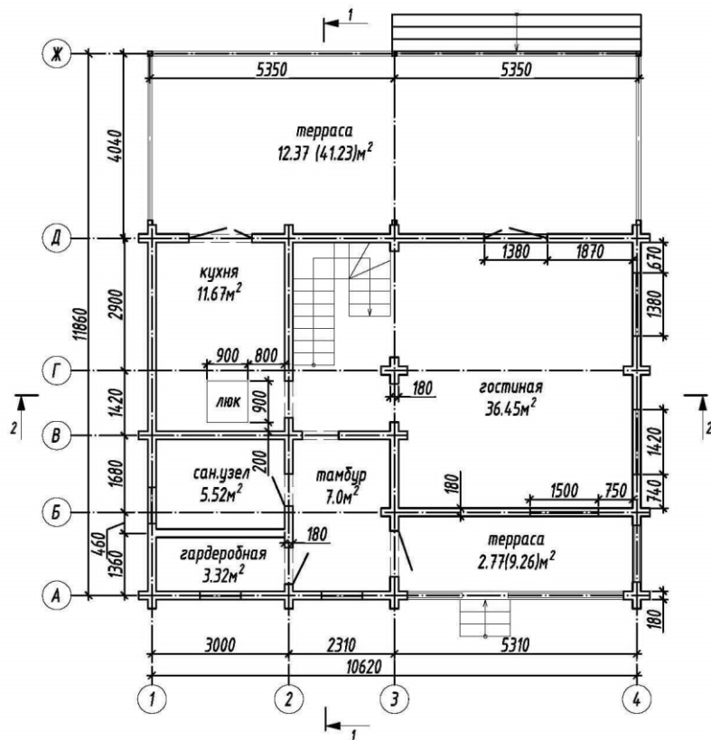
План 1 этажа
