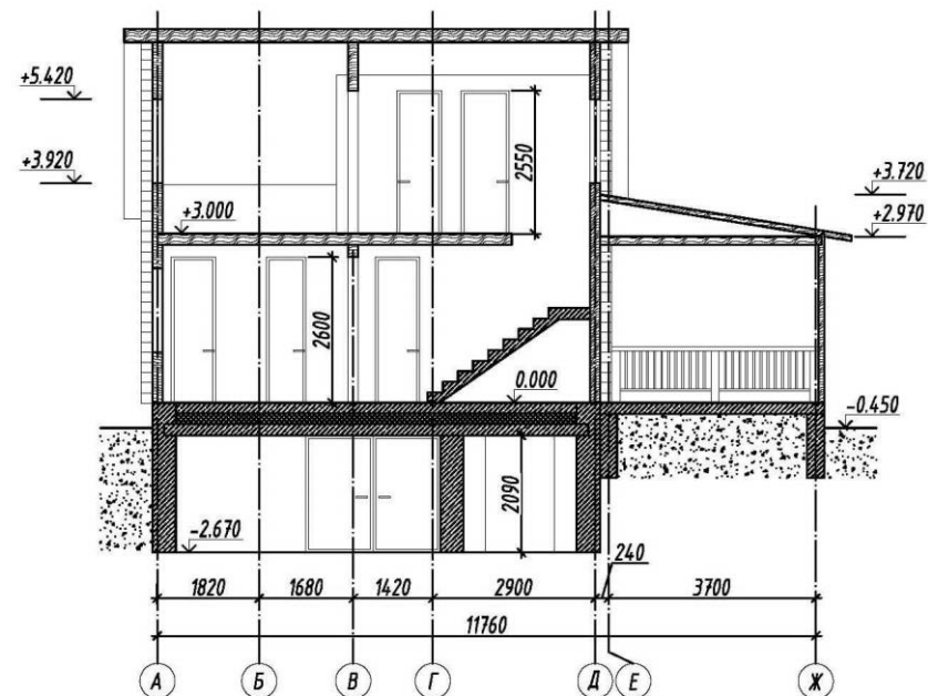
Разрез 1-1
